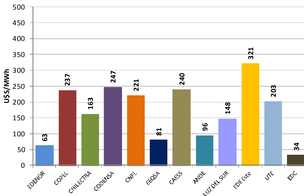
Tarifa Eléctrica - Cliente Comercial Cef 10 kW - 2.000 kWh/mes - BT DICIEMBRE/2011
