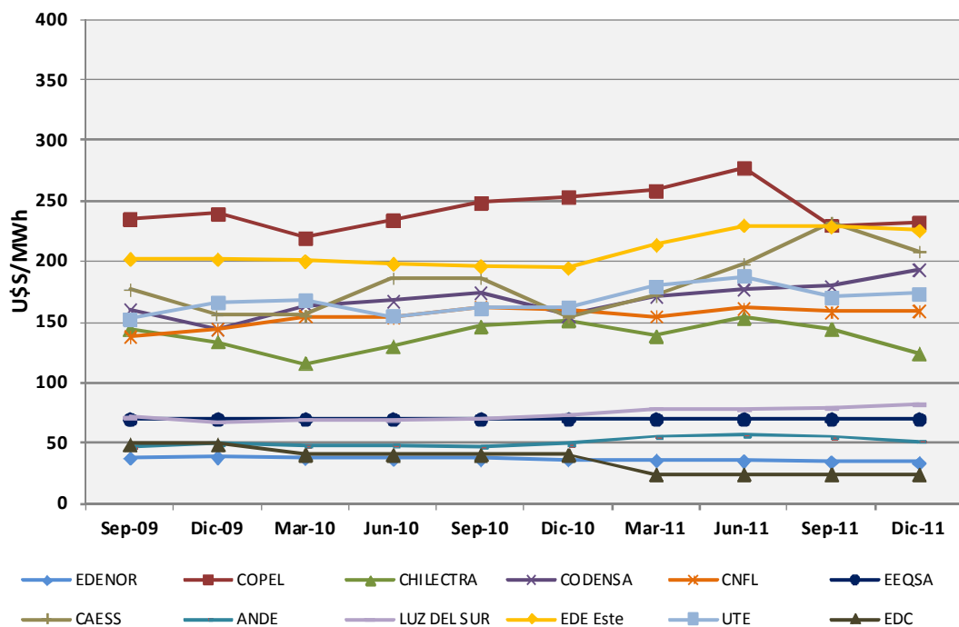
Evolución de la tarifa industrial con impuestos
