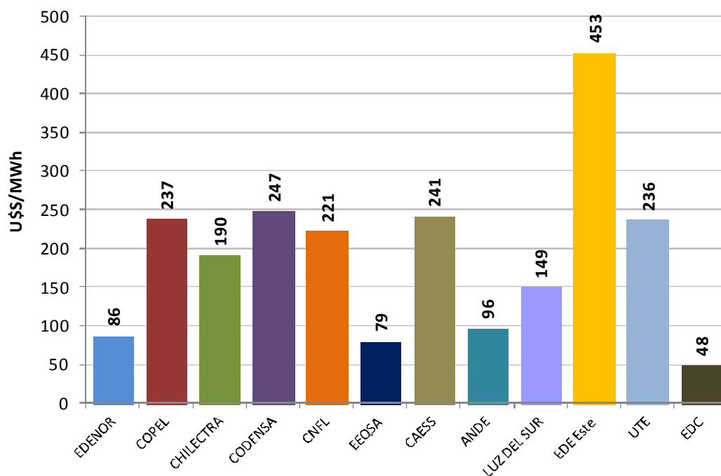
Tarifa Eléctrica - Cliente Comercial Cd 10 kW - 1.000 kWh/mes - BT DICIEMBRE/2011
