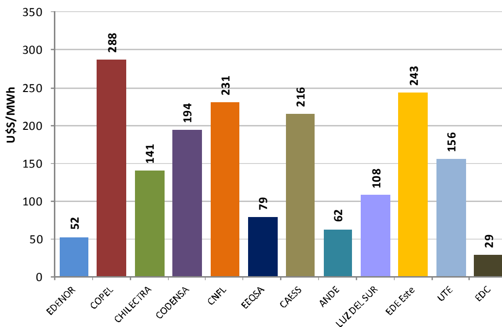
Tarifa Eléctrica - Cliente Industrial If 300 kW - 50.000 kWh/mes - MT DICIEMBRE/2011
