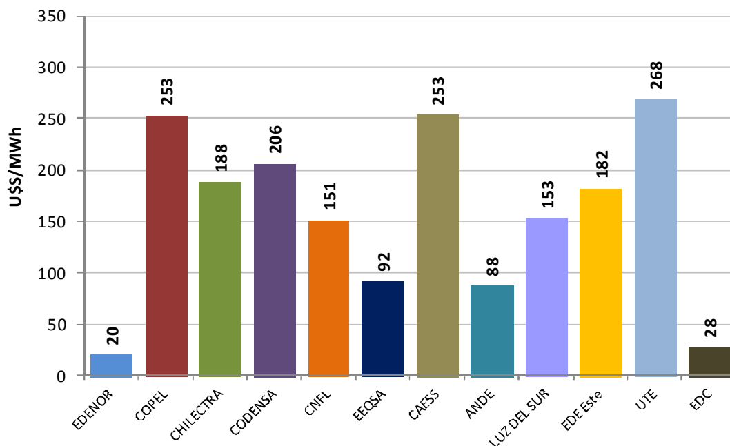
Tarifa Eléctrica - Cliente Residencial Re Pot. Mínima Admitida - 400 kWh/mes - BT DICIEMBRE/2011
