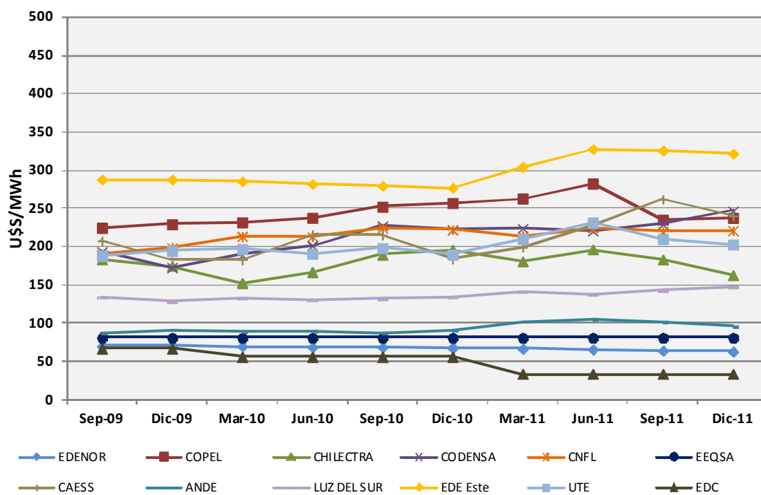
Evolución de la tarifa comercial con impuestos
